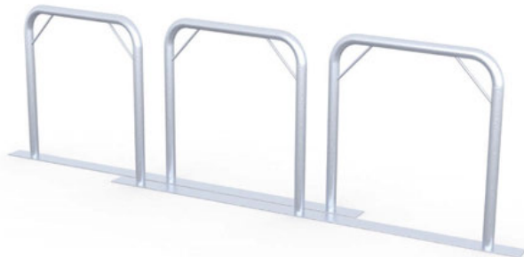
ARIS MOBIL Element mit 3 Bügeln verzinkt zusammengelegt für den Transport oder zur Lageraufbewahrung.
