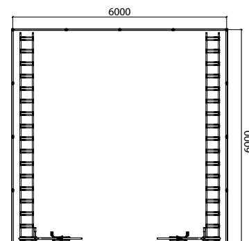
Draufsicht Modul 3, 4 x 4 Felder, 34 Fahrräder
