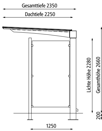
Seitenansicht einseitig mit Seitenwand
