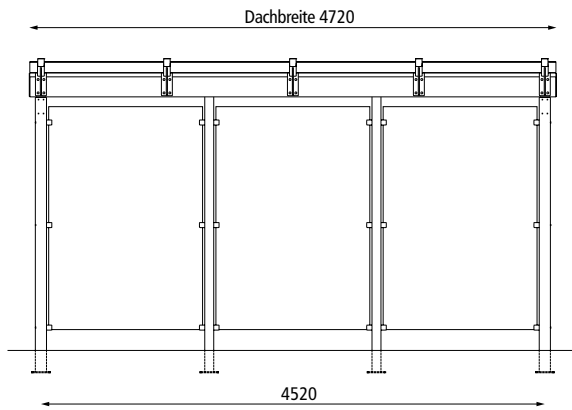
Frontansicht mit Rückwand, Modul 1
