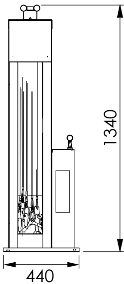
Frontansicht
