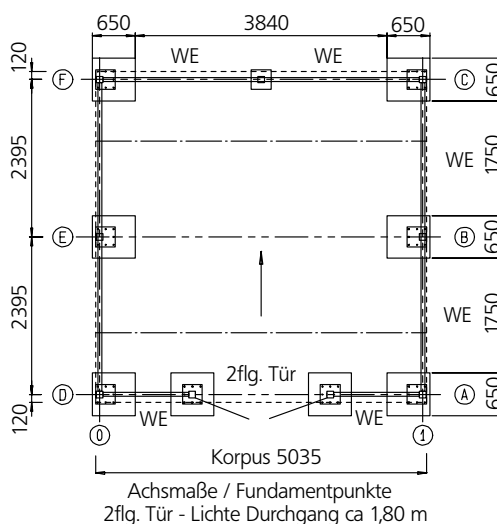
Modul 4, Draufsicht
