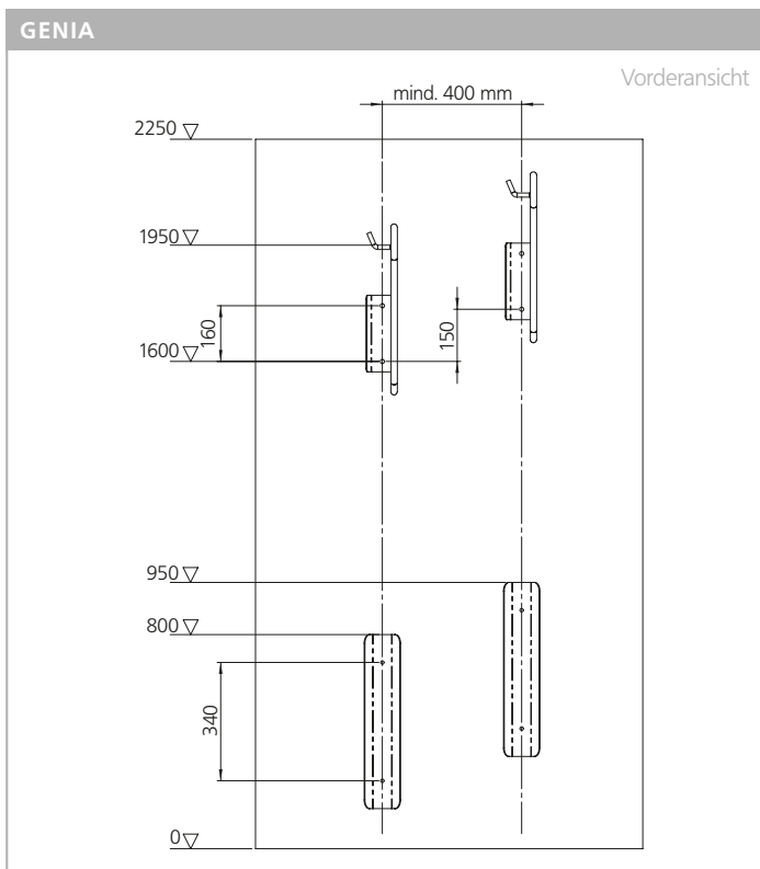
GENIA Einzelparker verzinkt zur Wandmontage.
