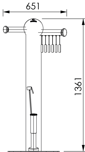
Frontansicht
